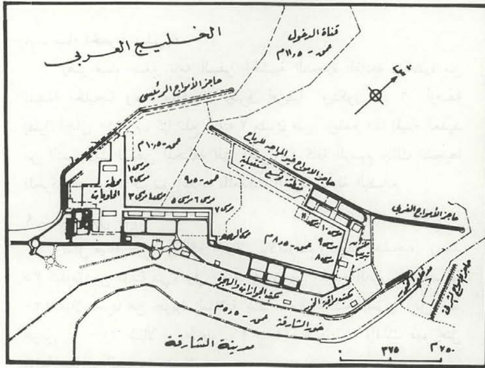
شکل رقم (۵) مخطط ميناء خالد
