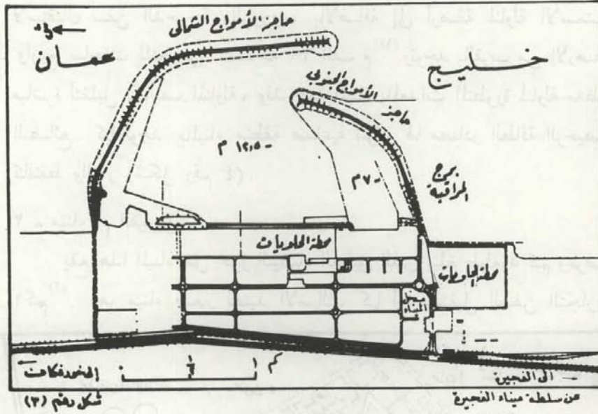
مخطط ميناء الفجيرة
