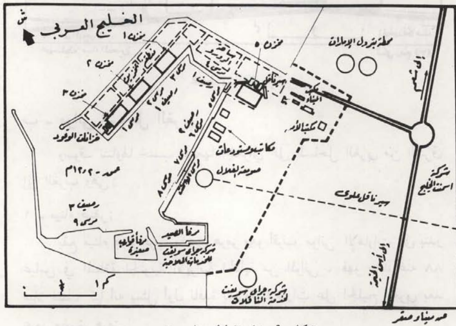
شكل رقم (٤) خطط ميناء صقر
