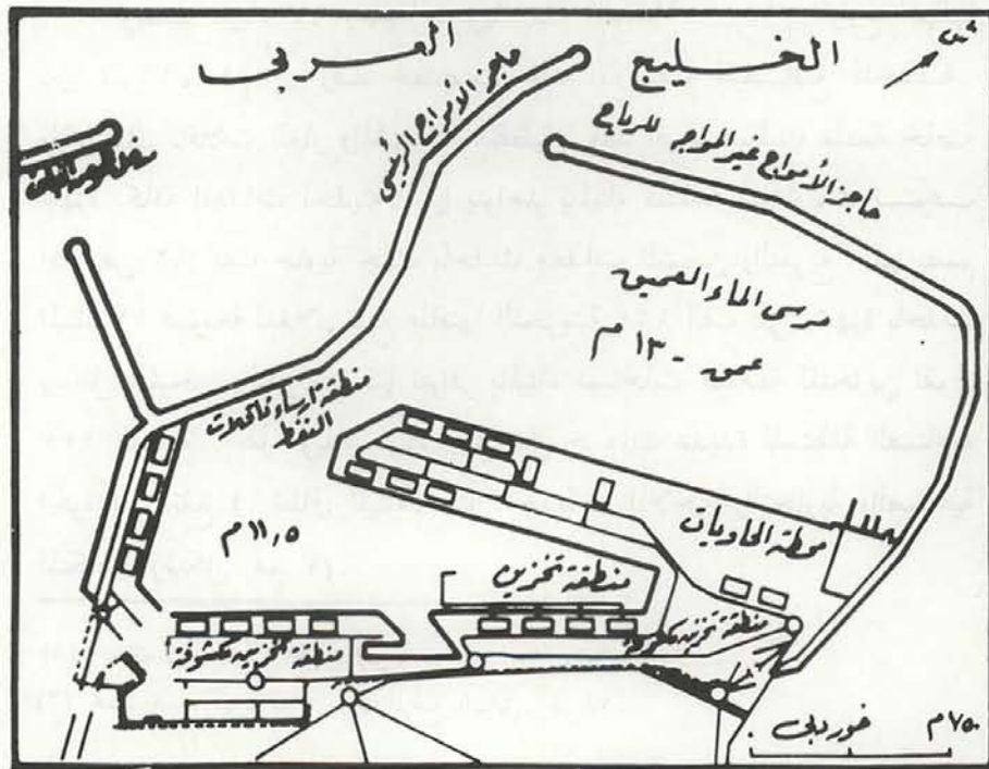
شکل رقم (۶) مخطط ميناء راشد
